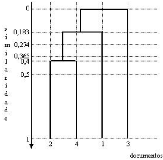
FIG. 3.8: Resultado do método de ligação completa
