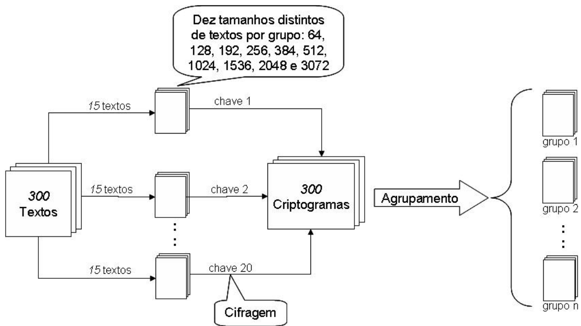
FIG. 5.5: Fluxograma para execução do 3º experimento
