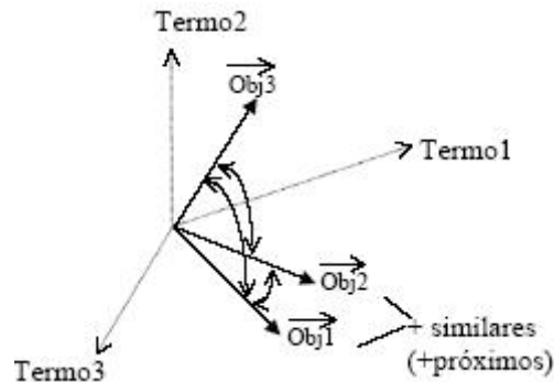
FIG. 3.2: Modelo de espaço vetorial
