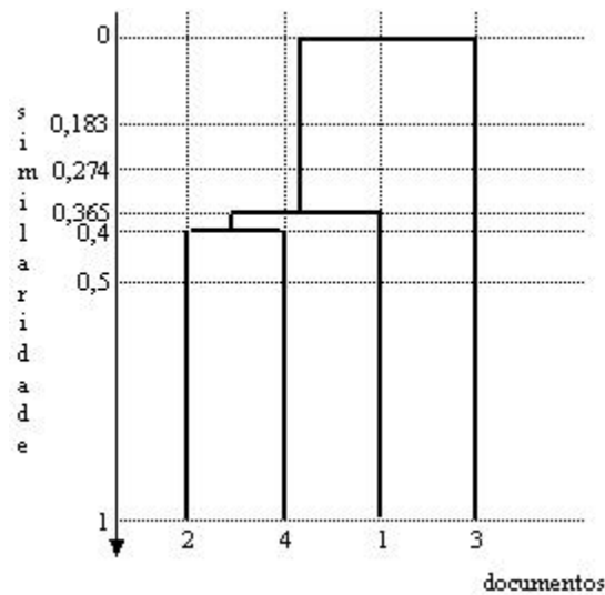
FIG. 3.6: Resultado do método de ligação simples
