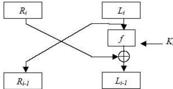
FIG. 2.4: Estrutura de Feistel para decifrar ( i = r, r - 1, \dots, 1 )
