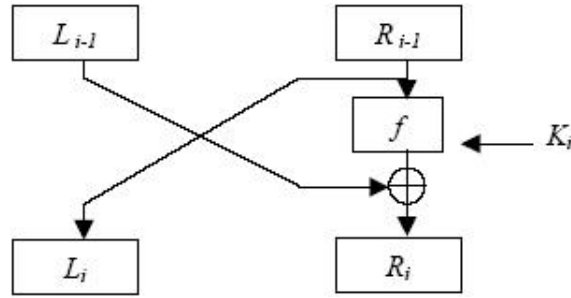
FIG. 2.3: Estrutura de Feistel para cifrar ( i = 1, 2, \dots, r )
