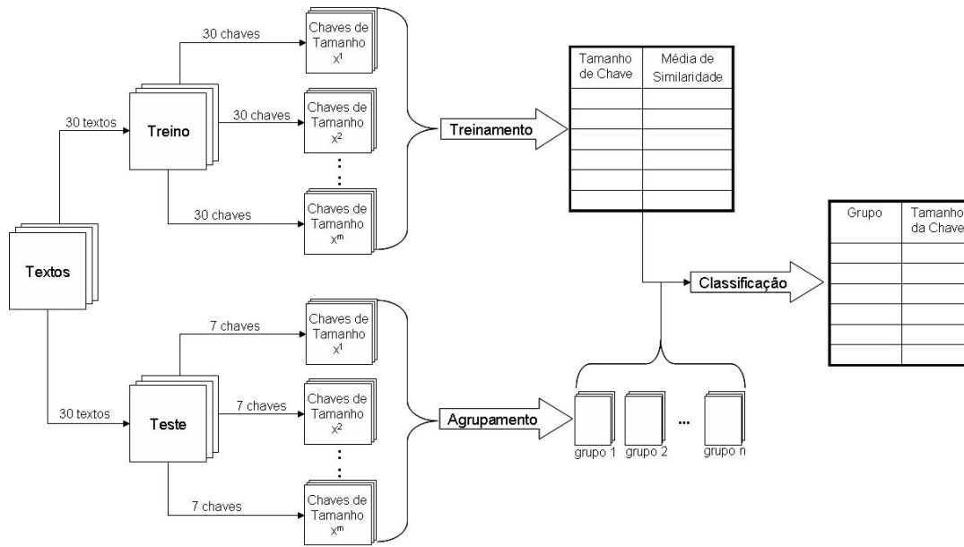
FIG. 4.1: Fluxograma do treinamento e validação do procedimento de determinação do período da chave
