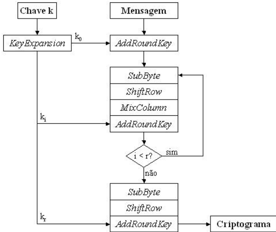
FIG. 2.6: Fluxograma do AES
