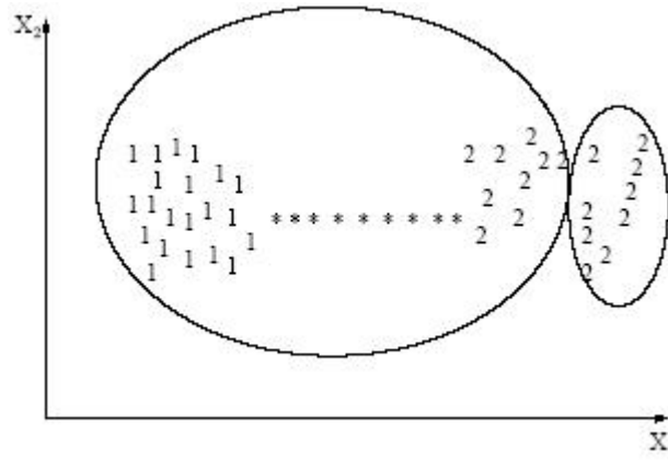
FIG. 3.5: Efeito do método de ligação simples em um ambiente esférico
