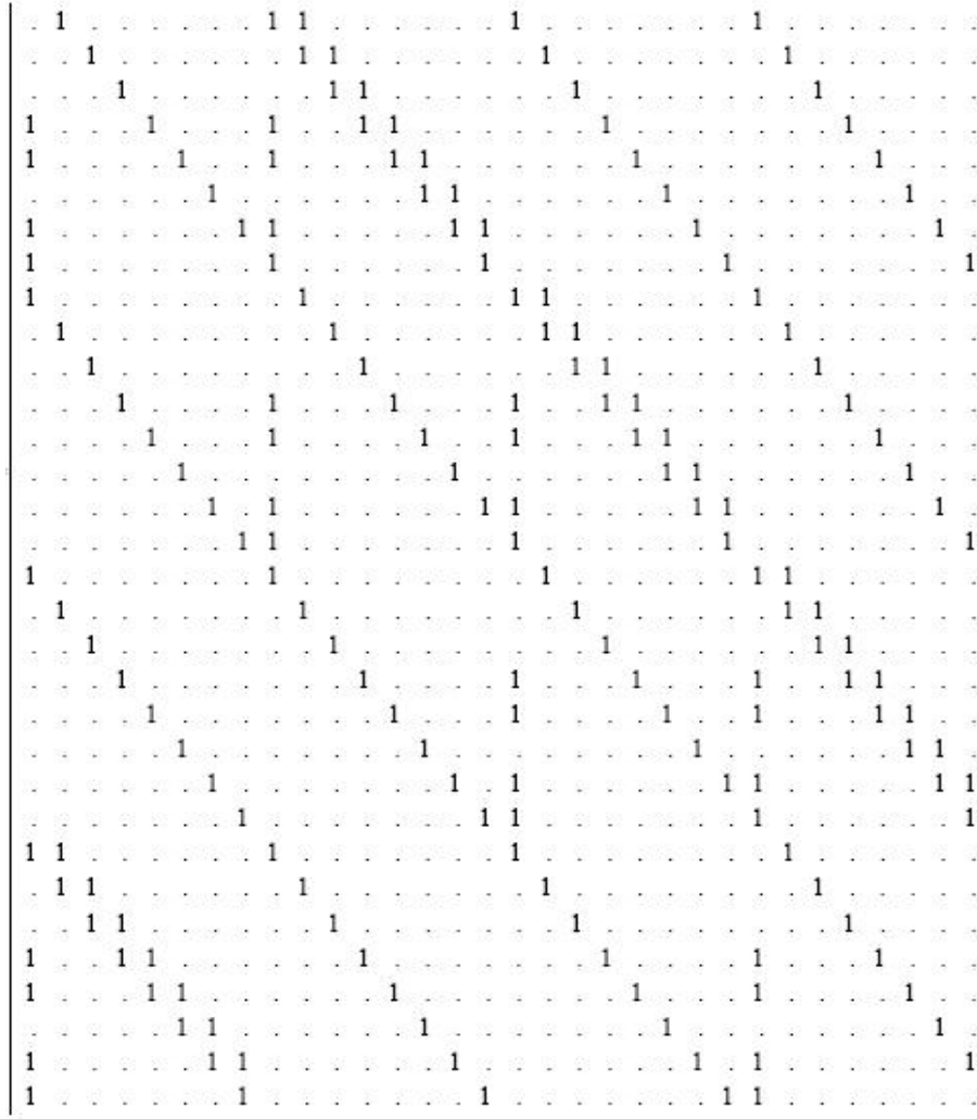
FIG. 2.7: Ilustração da matriz M_{32 \times 32} (Obs: '.' = 0 )
