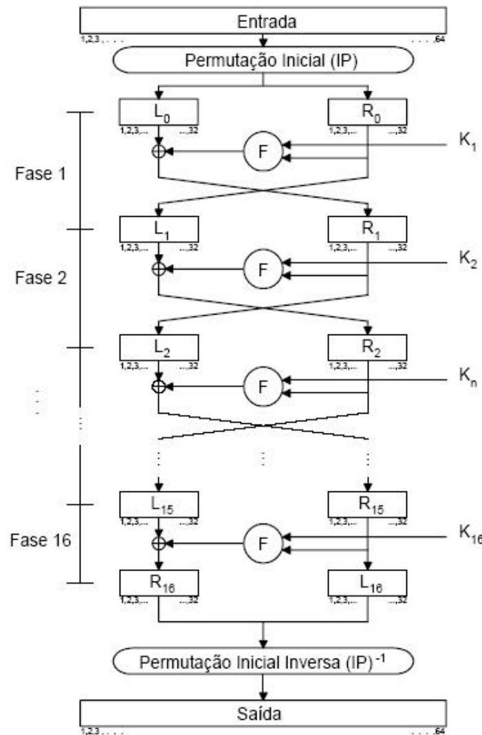
FIG. 2.5: Fluxograma do DES
