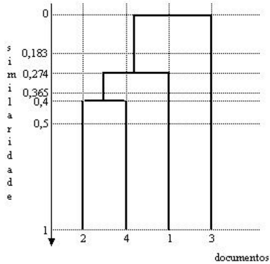
FIG. 3.9: Resultado do método de ligação por média dos grupos
