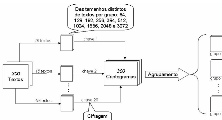
FIG. 6.7: Descrição do segundo conjunto de experimentos (CARVALHO, 2006)
