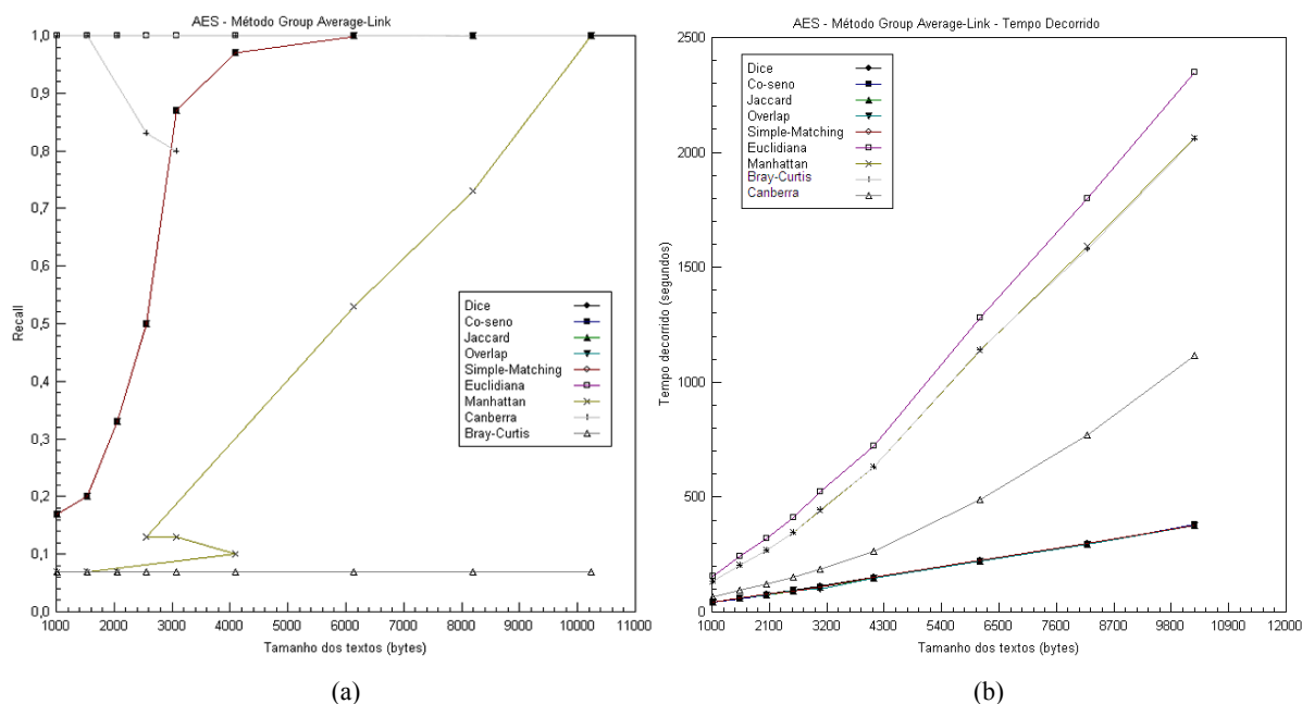
GRA. 6.10: Recall e tempo decorrido para o algoritmo AES, com chaves de 128 bits , com o método Group Average-Link
