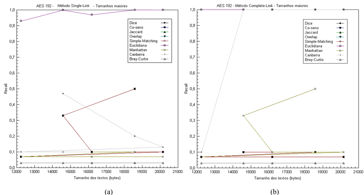
GRA. 6.17: Recall para o algoritmo AES, com chaves de 192 bits , com os métodos Single-Link e Complete-Link
