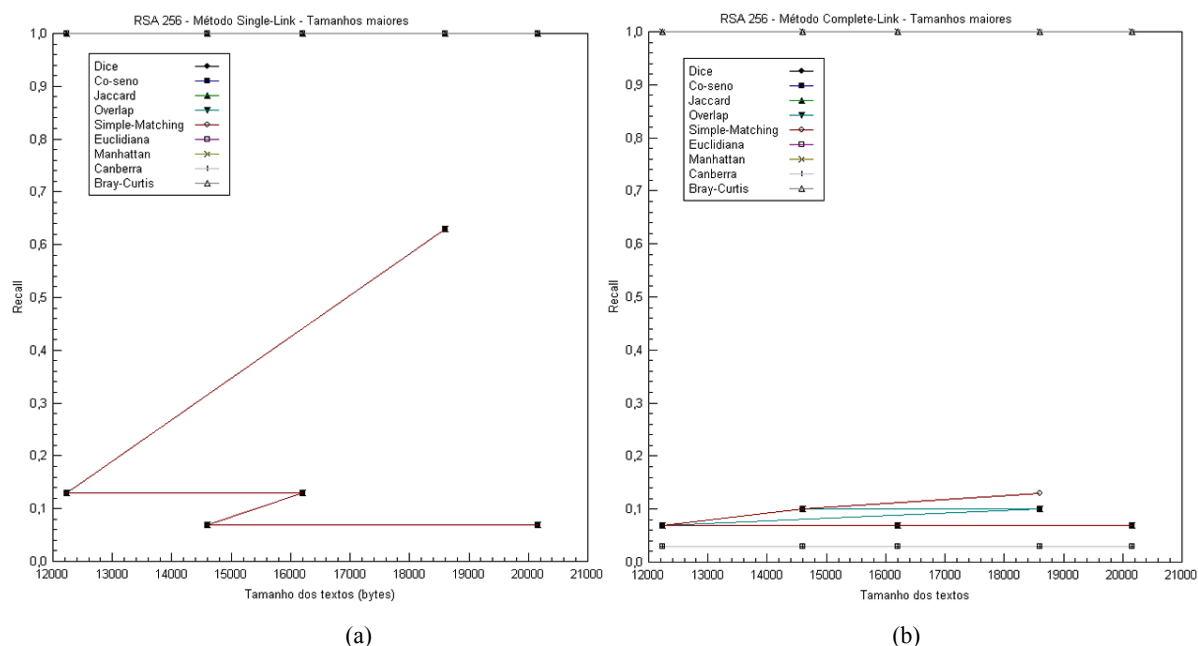
GRA. 6.19: Recall para o algoritmo RSA, com chaves de 256 bits , com os métodos Single-Link e Complete-Link
