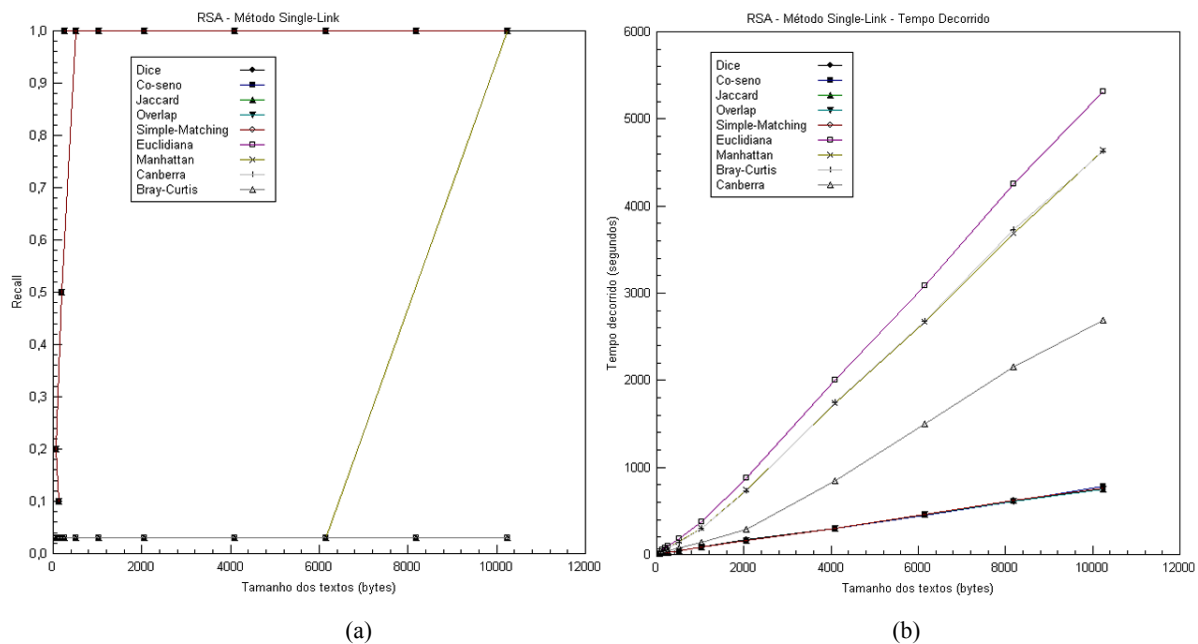
GRA. 6.11: Recall e tempo decorrido para o algoritmo RSA com, com chaves de 64 bits, com o método Single-Link
