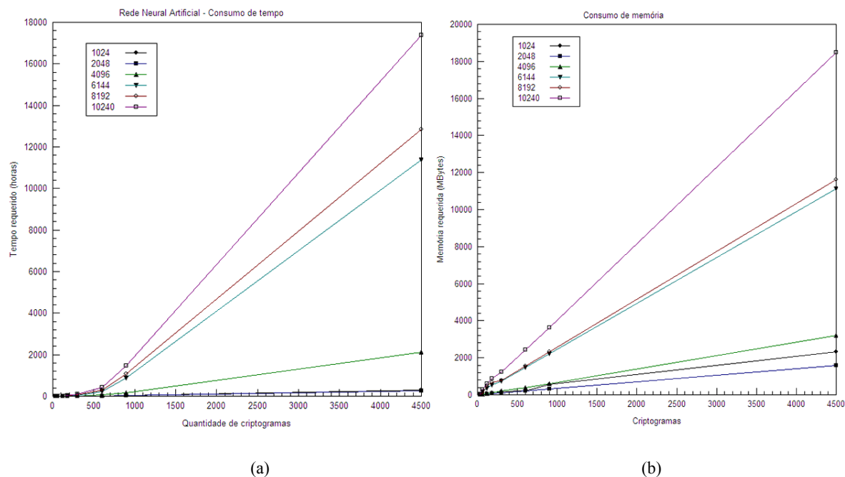
GRA. 9.17.1: Tempo de execução e necessidade de memória para a rede neural artificial
