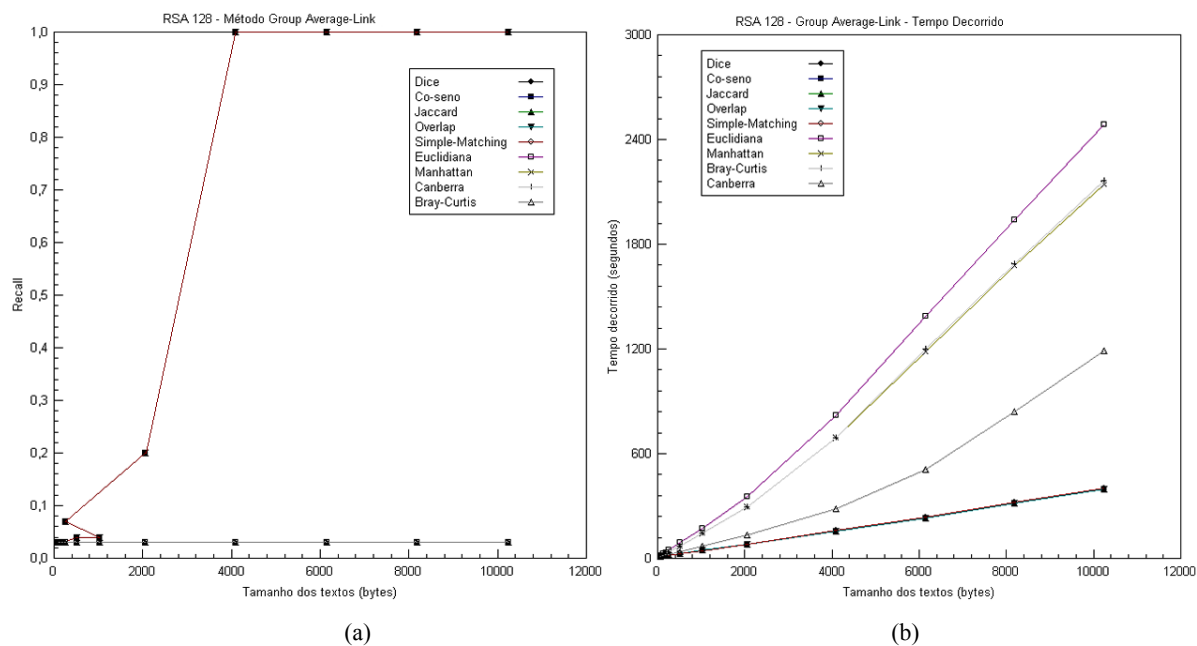
GRA. 6.16: Recall e tempo decorrido para o algoritmo RSA com, com chaves de 128 bits , com o método Group Average-Link
