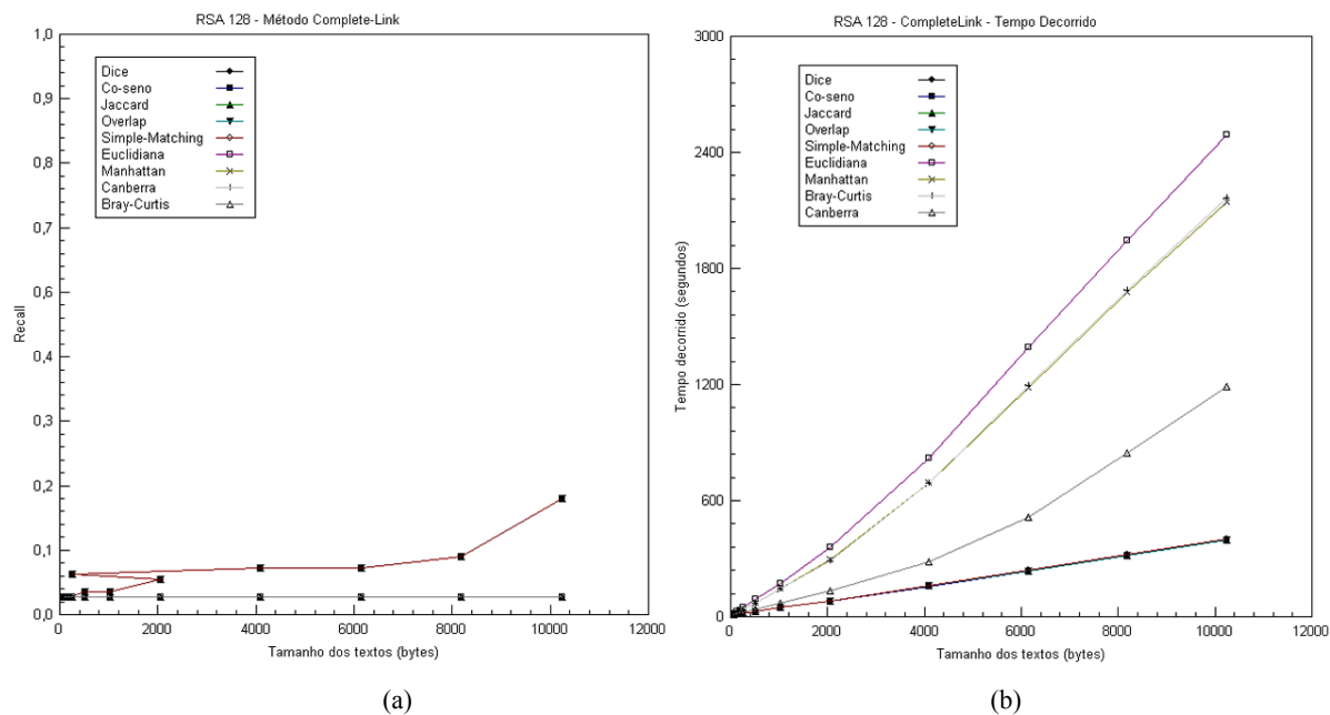
GRA. 6.15: Recall e tempo decorrido para o algoritmo RSA com, com chaves de 128 bits , com o método Complete-Link
