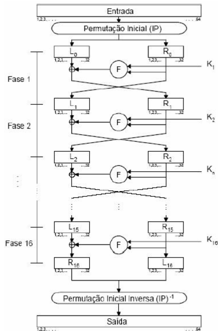
FIG. 2.9: Descrição do funcionamento do DES (CARVALHO, 2006)
