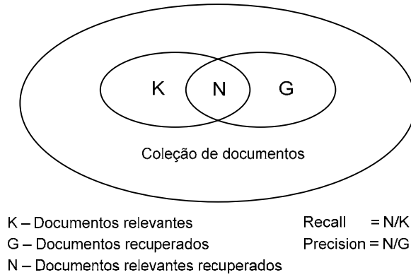
FIG. 3.13: Precision e recall
