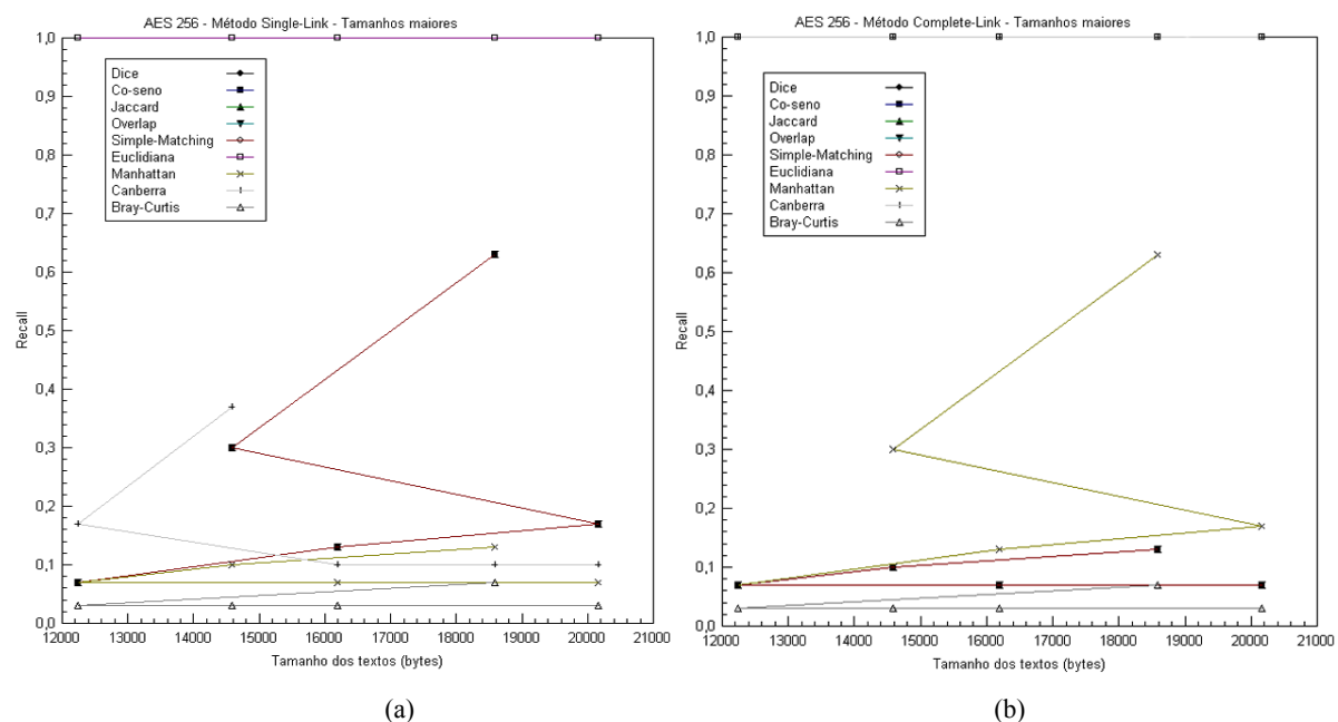
GRA. 6.18: Recall para o algoritmo AES, com chaves de 256 bits , com os métodos Single-Link e Complete-Link
