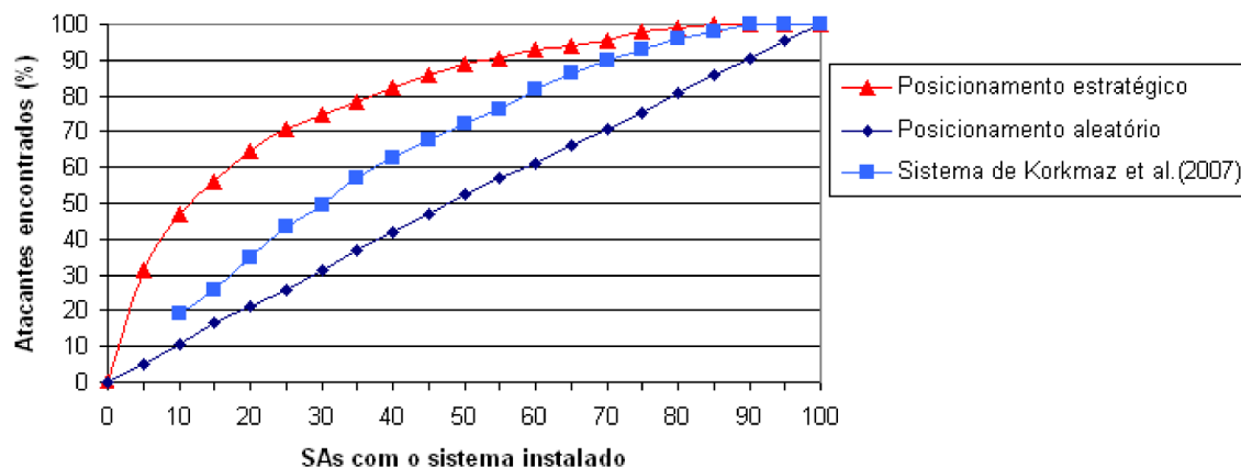
FIG. 5.11: Comparação de eficiência: Sistema proposto x Sistema de Korkmaz et al. (KORKMAZ, 2007).
