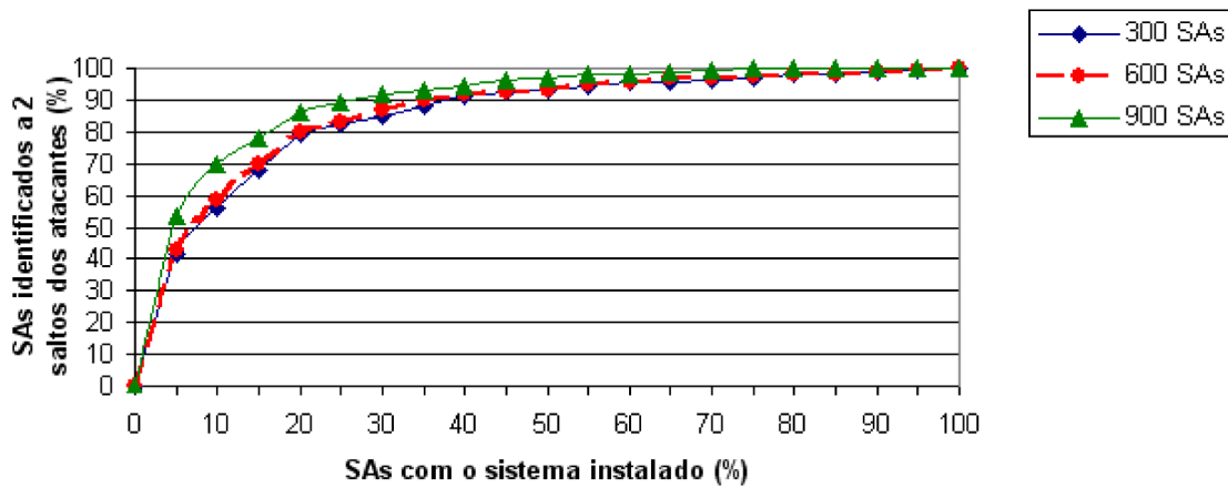
FIG. 5.5: Quantidade de SAs identificados a 2 saltos dos atacantes - Posicionamento estratégico.
