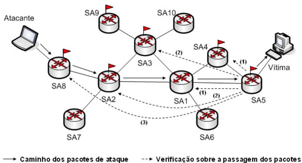
FIG. 3.4: Sistema de Korkmaz et al. (KORKMAZ, 2005).
