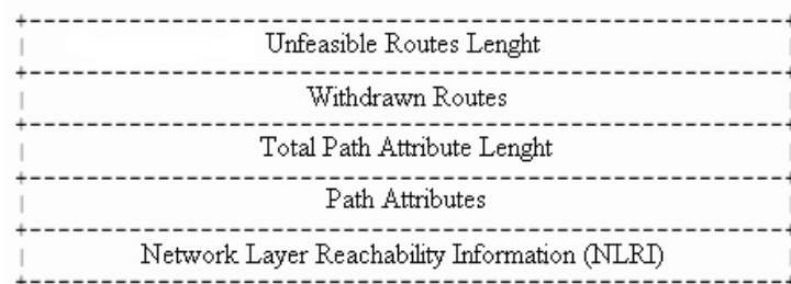
FIG. 4.4: Formato da mensagem Update.
