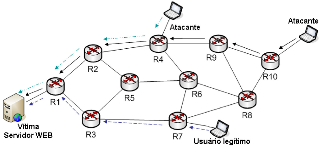
FIG. 1.1: Exemplo de utilidade do rastreamento de tráfego.
